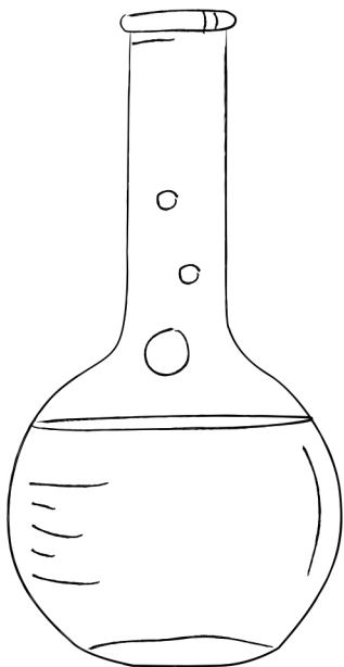
Der Rundkolben
