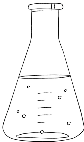
Der Erlenmeyerkolben
