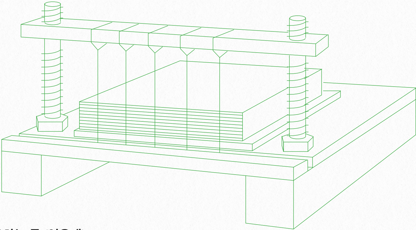
책을 실로 엮을때 사용하는 틀 (엮음대)
